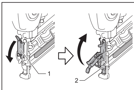
► 1. Latch 2. Door
